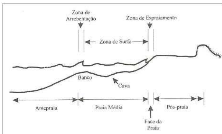
Figura 3.8 – Zonagem hidrodinâmica e morfológica numa praia oceânica. (Fonte: HOEFEL, 1998.)
