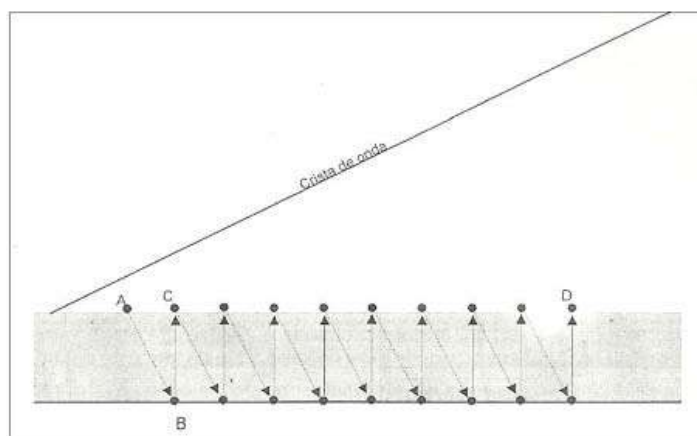
Figura 3.13 – Padrão de transporte em zig-zag. (Fonte: SILVA, et al., 2004.)
