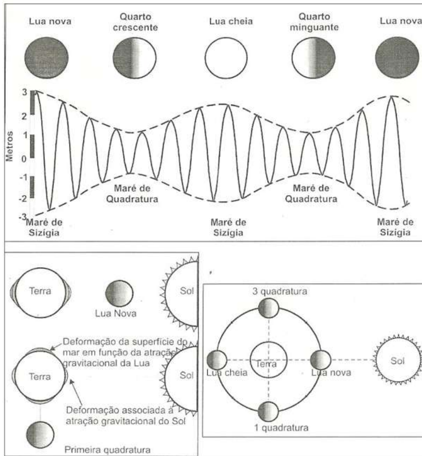
Figura 3.15 Ciclos de maré de sizígia e quadratura associados às fases de lua cheia, lua nova, quarto crescente e quarto minguante. (Fonte: Fonte: SILVA, et al., 2004.)
